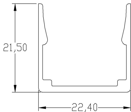
安装卡扣尺寸图
